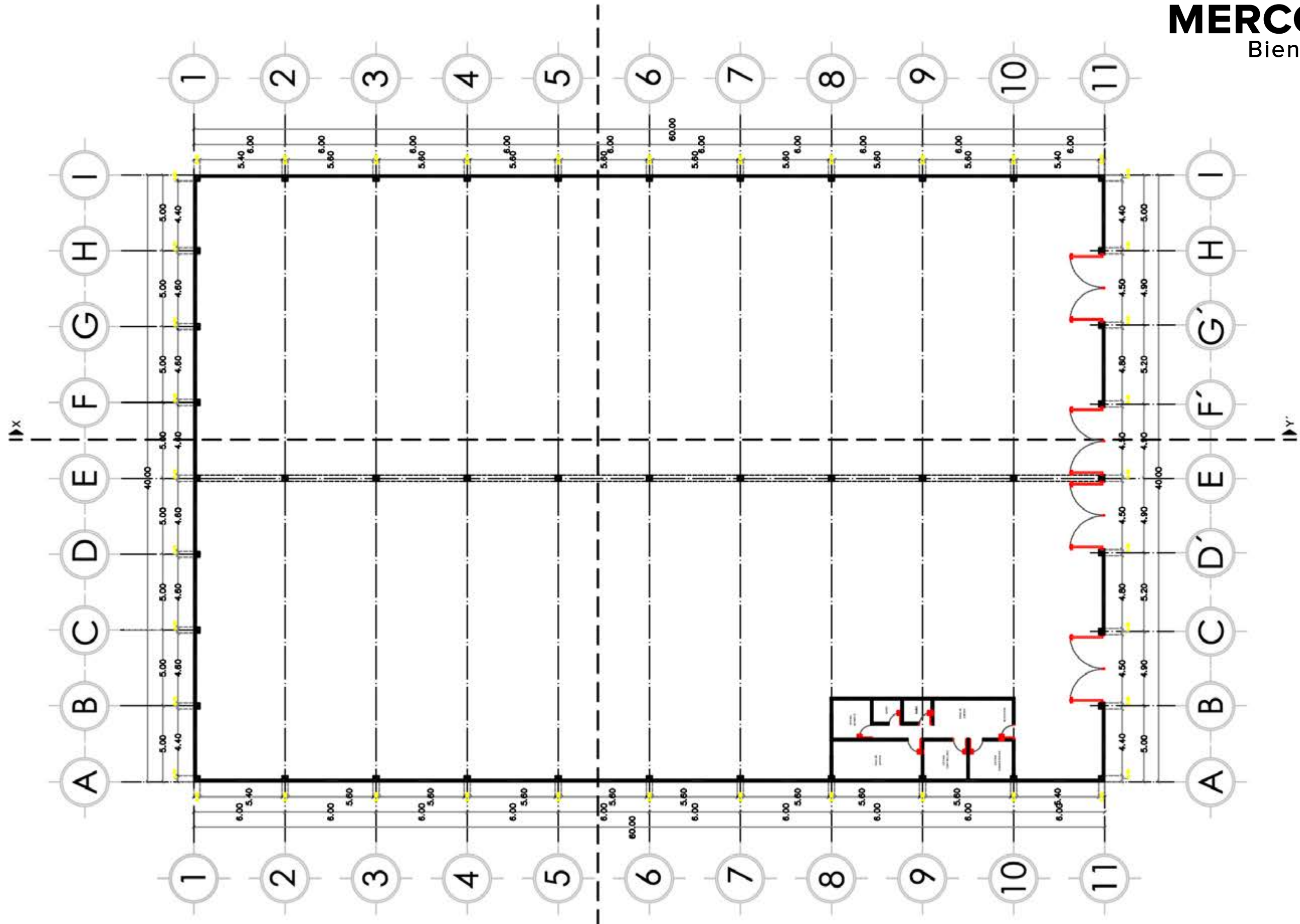
PLANTA ARQUITECTÓNICA
