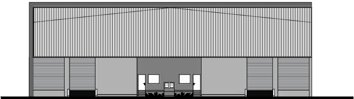
FACHADA
