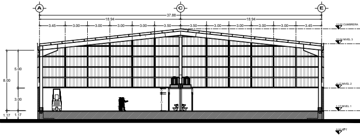
CORTE A-A'
