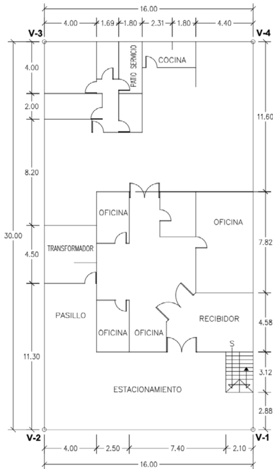
PLANTA ARQUITECTONICA B A J A
