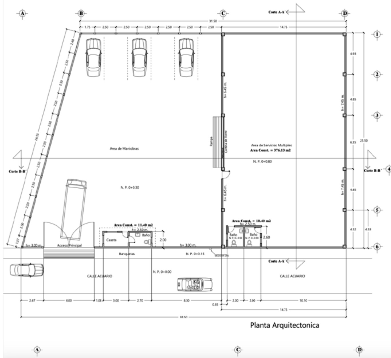
PLANTA BAJA ARQUITECTONICA
