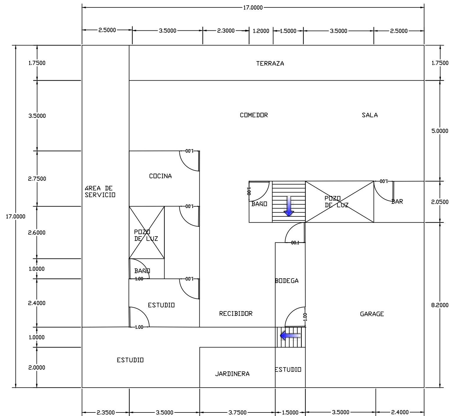
PLANTA BAJA Sup. 206.68 m2
