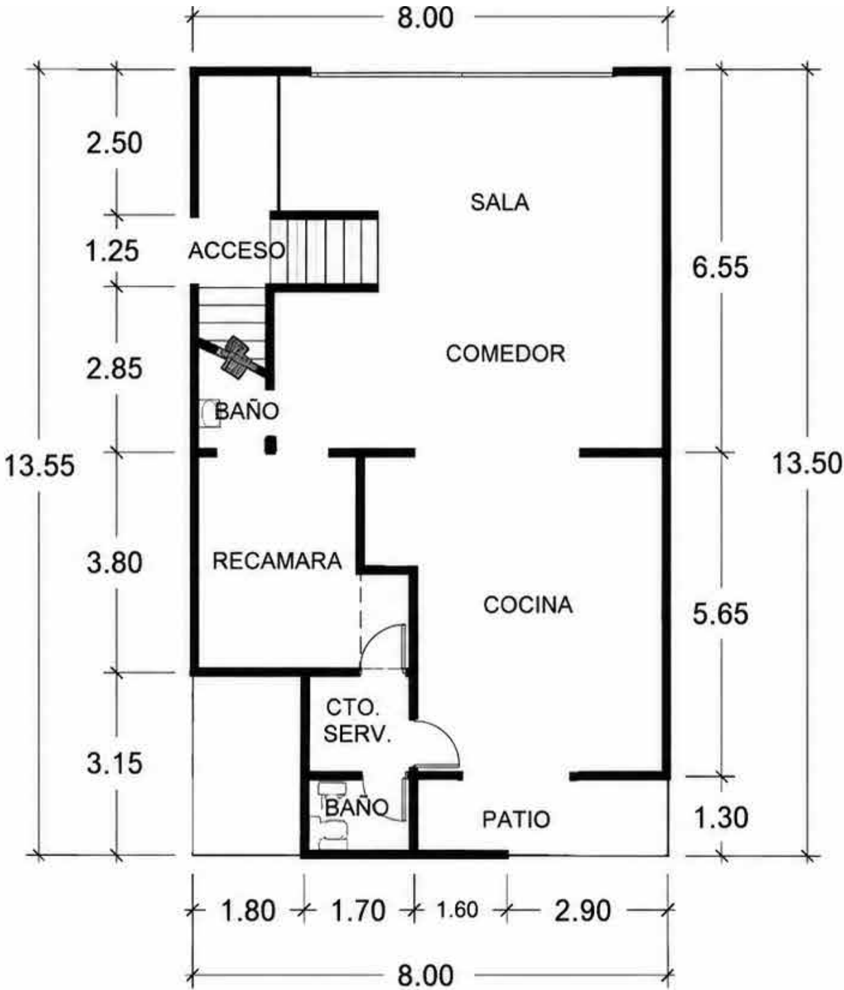
PLANTA BAJA SUP. 100.23 m 2
