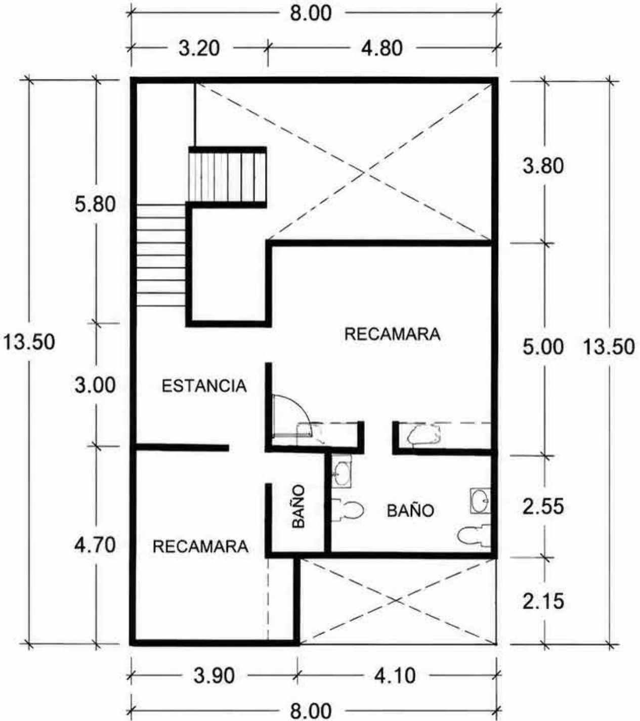
PLANTA ALTA SUP. 71.94 m²
