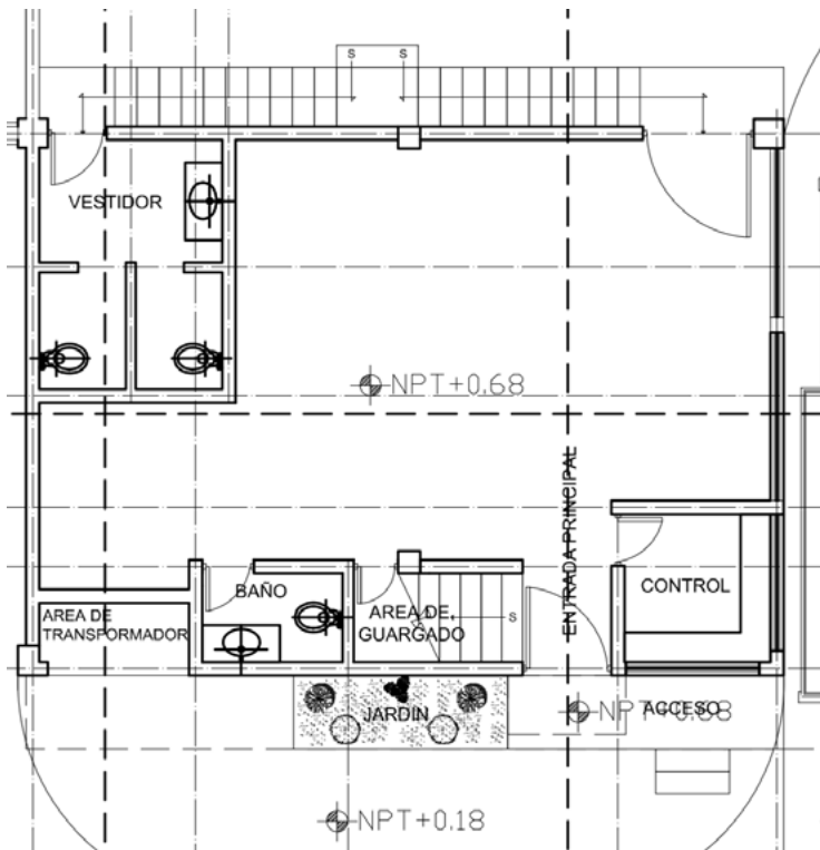
PLANO OFICINA
