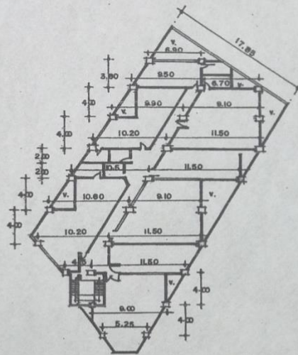
PLANTA ALTA ESC. 1: 500
