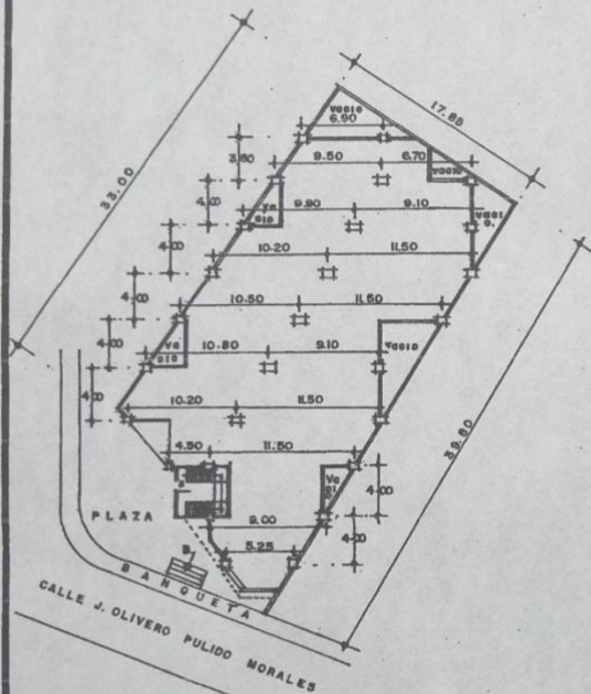
PLANTA BAJA Esc. 1: 500
